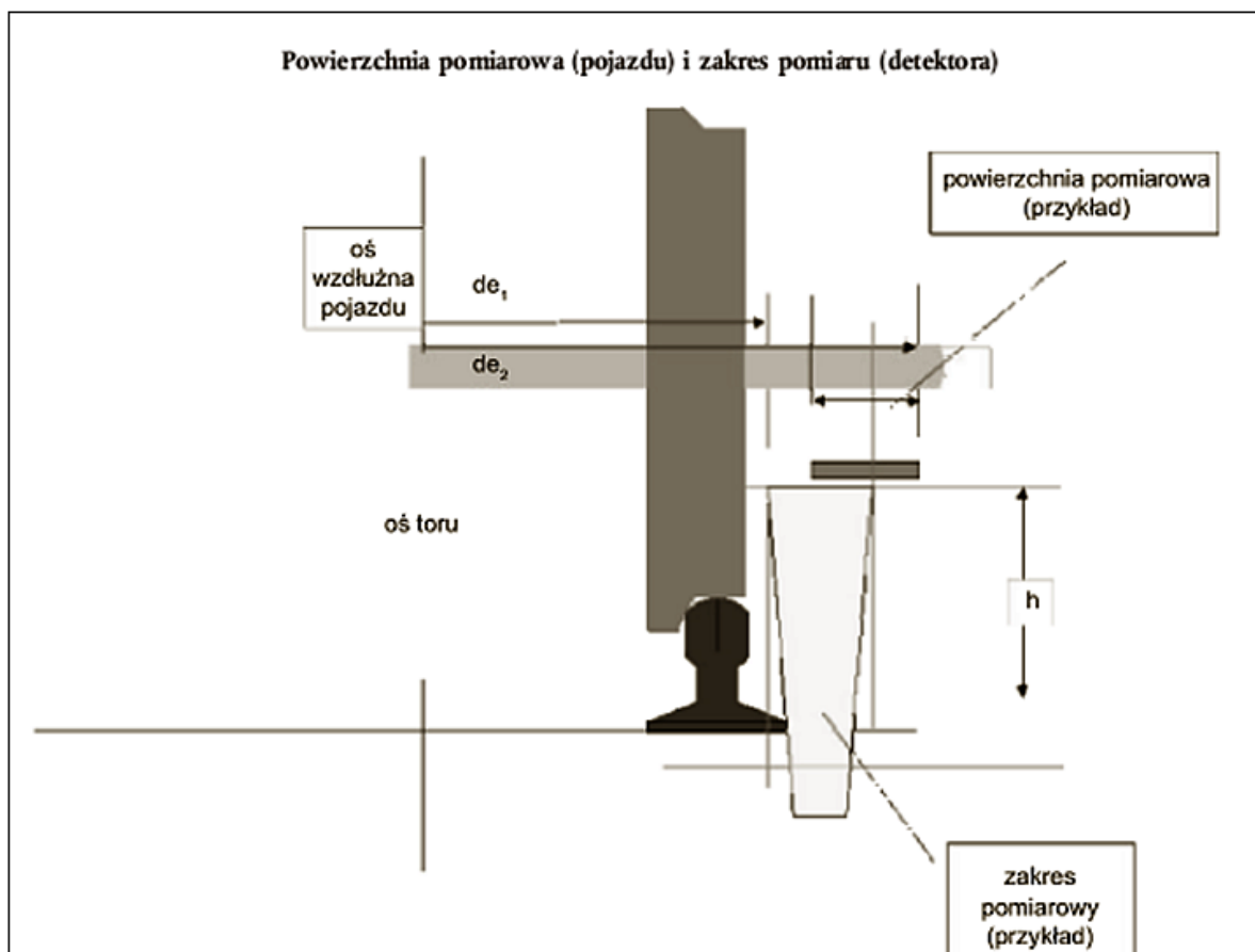
Rys. 1. Powierzchnia pomiarowa pojazdu i zakres pomiaru detektora wg. normy PN-EN 15437-1:2009
