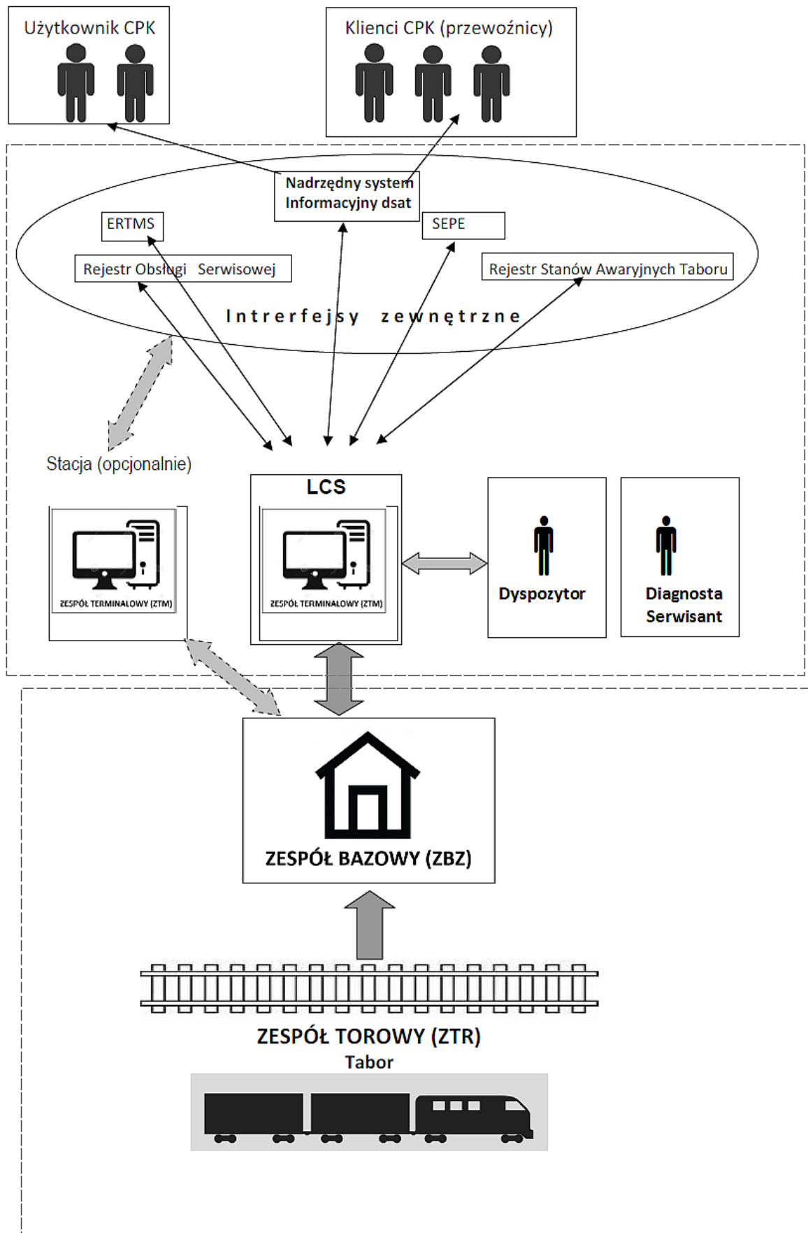
Rys.2. Architektura systemu dsat
